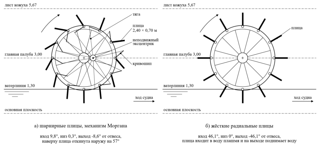
Колесо с шарнирными плицами и с жёсткими
