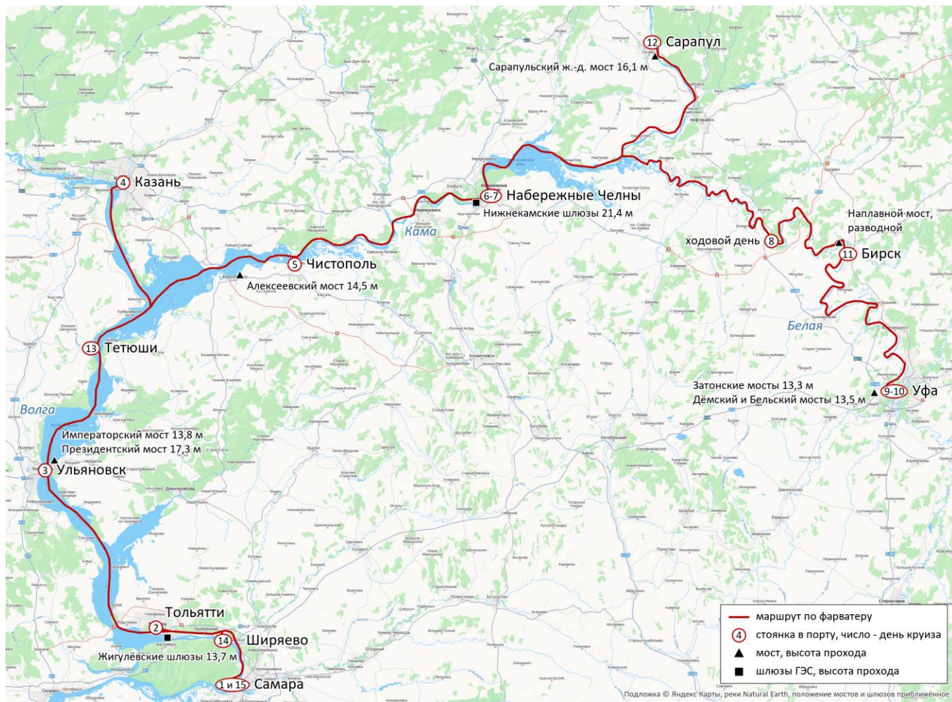
Маршрут по фарватеру, мосты и шлюзы
