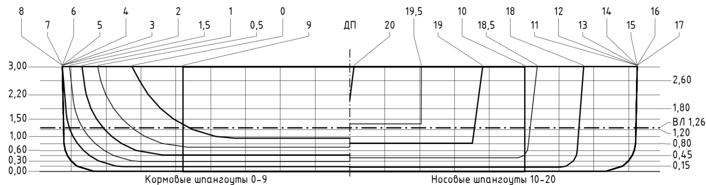
Обводы - шпангоуты корпуса и ватерлиния 1,26 м
